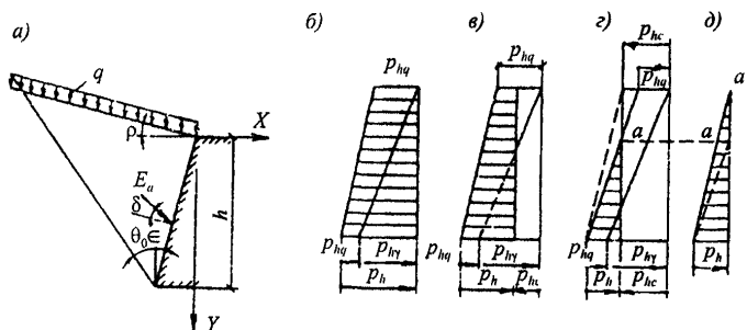
a – на стену; б – при отсутствии сцепления p_{hc} = 0 ; в – при p_{hc} < p_{hq} ; г – при p_{hc} \geq p_{hq} ; д – заменяющая (расчетная) эпюра
