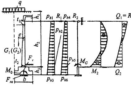
Рисунок 3 – Расчетная схема стены подвала
